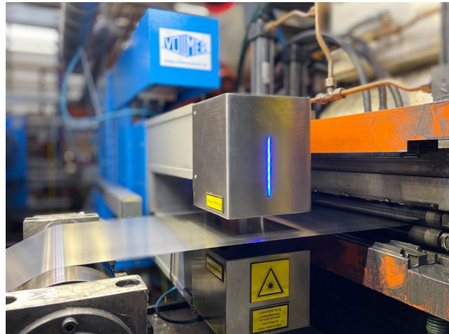
Eine neue Lasermessanlage ersetzt bei der MK Metallfolien GmbH das bestehende Isotopenmessverfahren zur Dickenmessung der Stahlbänder.
